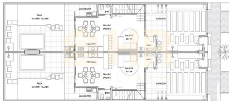
Planta baixa - Terreo
